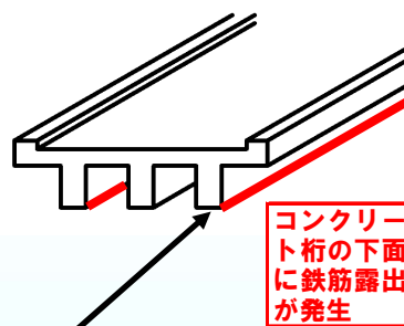
主桁の損傷（鉄筋露出）
