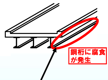
主桁の損傷（腐食）
