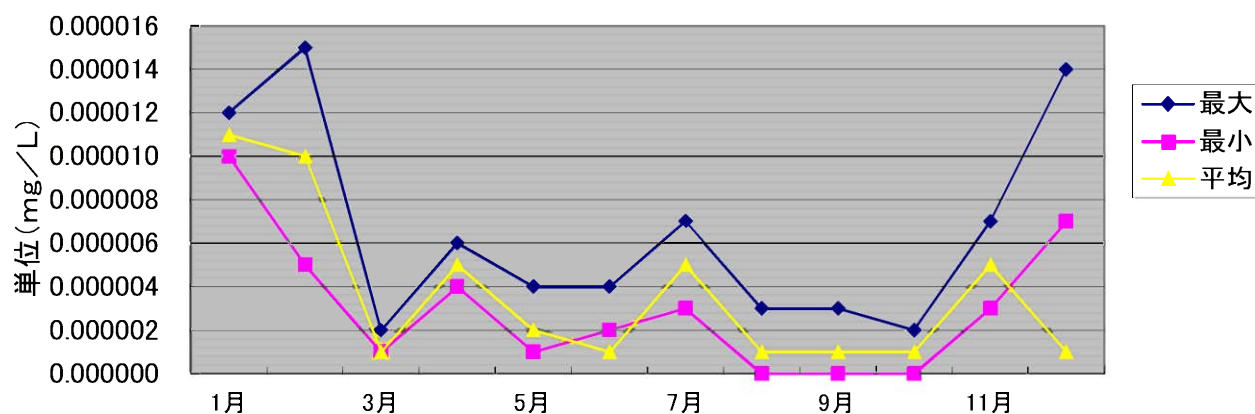
令和4年 カビ臭(2-MIB)の動向(原水)
