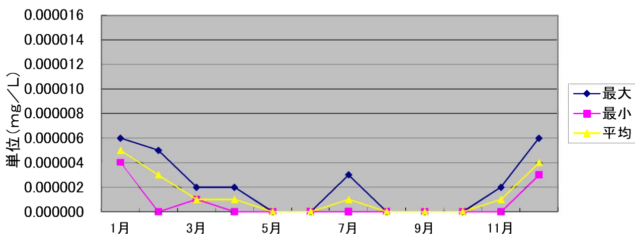
令和4年 カビ臭(2-MIB)の動向(浄水)
